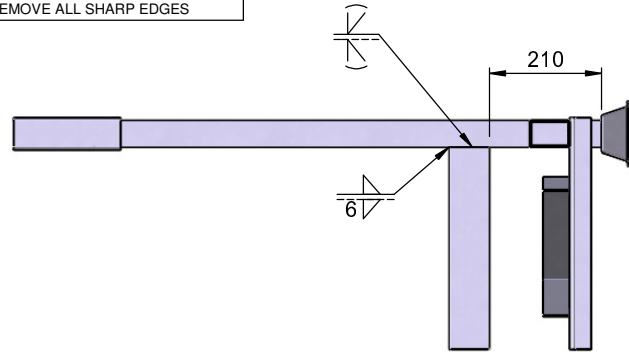
SECTION 1-1 SCALE 1 : 10
